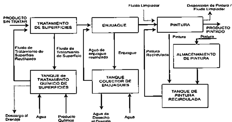
Figura No. 34: Esquema de flujo acabado final de pintura para efectos de una auditoria ambiental
